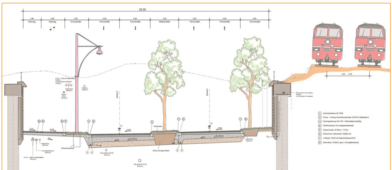
Regelquerschnitt Innerer Stadtring im Einschnittsbereich
